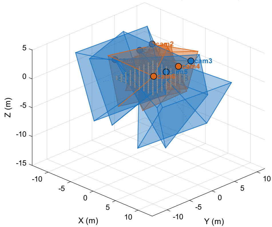
OptiTrack ad-hoc — 7 cams (Cost: 0.1449)
